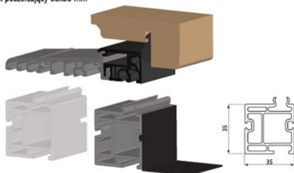
Element poszerzający 35x35 mm
